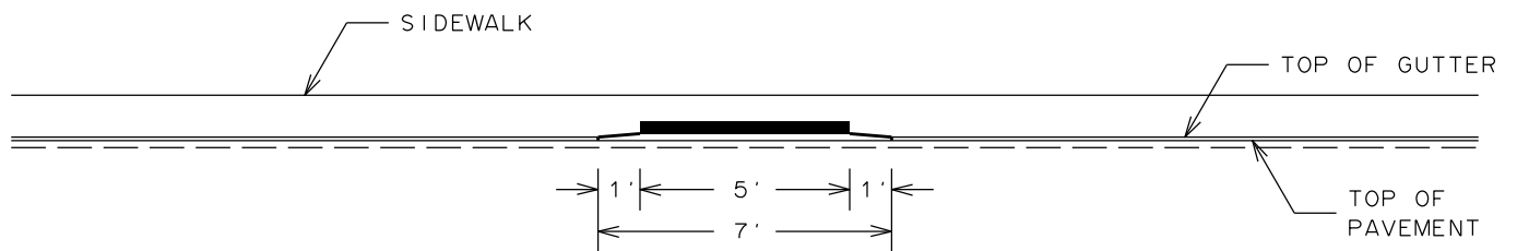
VIEW A-A
